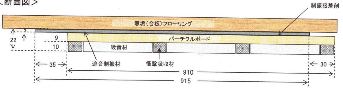
<断面図>
